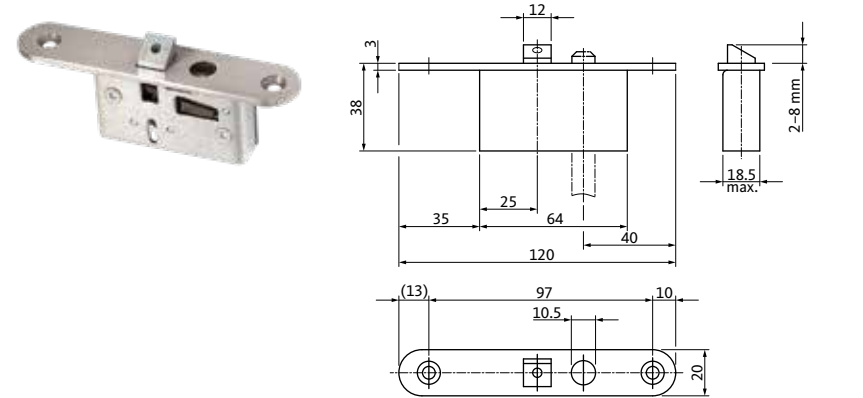
Schaltschloss B 1595 Stulpform: abgerundet/gerade
