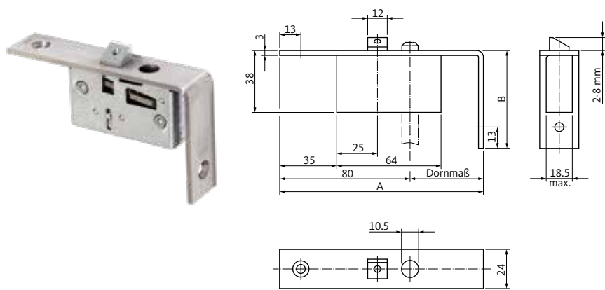
Schaltschloss B 1595 Stulpform: eckig/abgewinkelt
